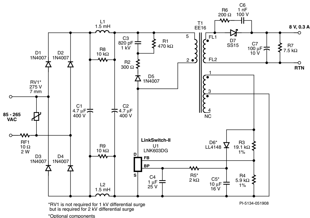
图 1. 2.4 W通用输入恒压 / 恒流充电器电源的电路图
